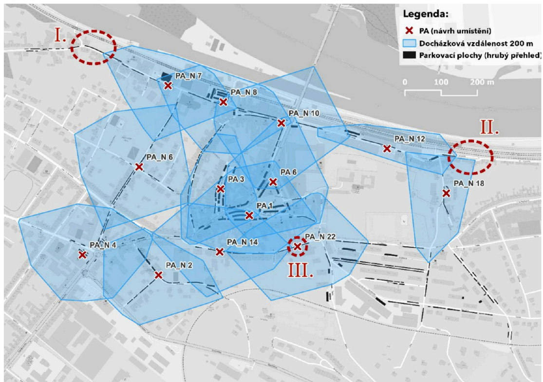
Obrázek 3.3: Návrh rozmístění PA a docházková vzdálenost 200 m.
