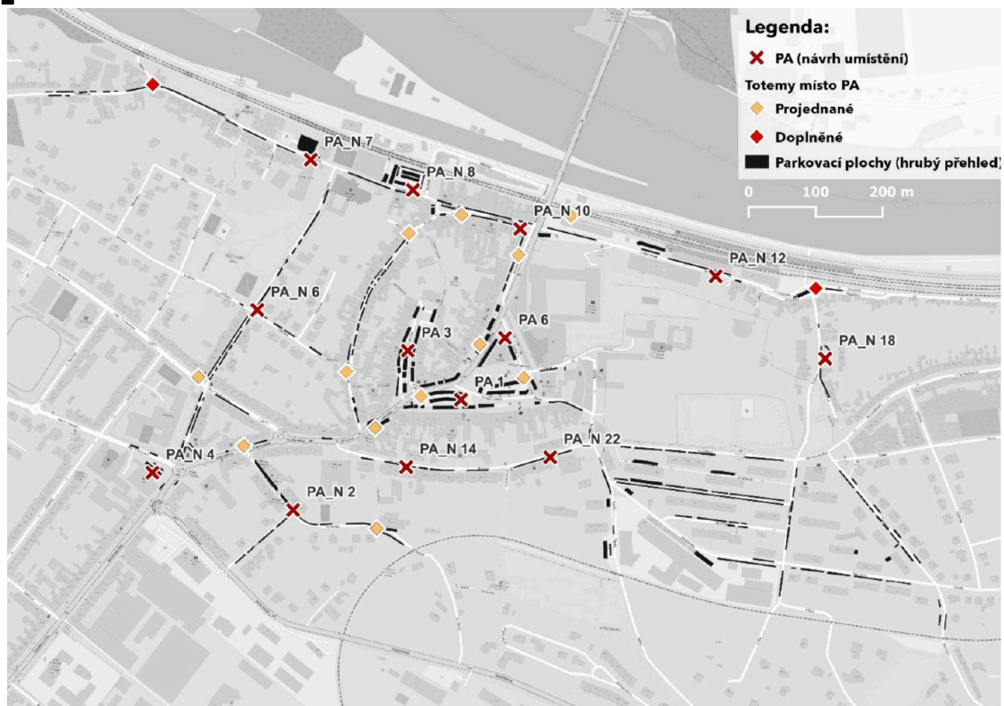
Obrázek 3.4: Návrh rozmístění PA a totemů pro stávající fázi.
